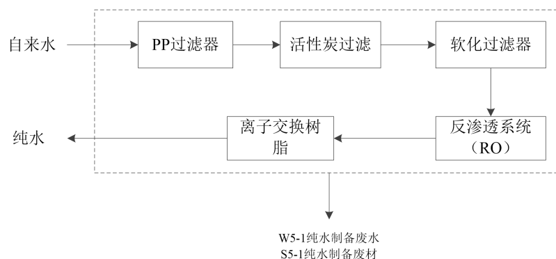
图 2-6 纯水制备工艺流程和产污环节示意图
